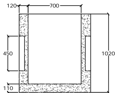
SECCION A-A
