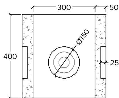
SECCION A-A
